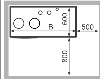
Kessel im Heizraum
