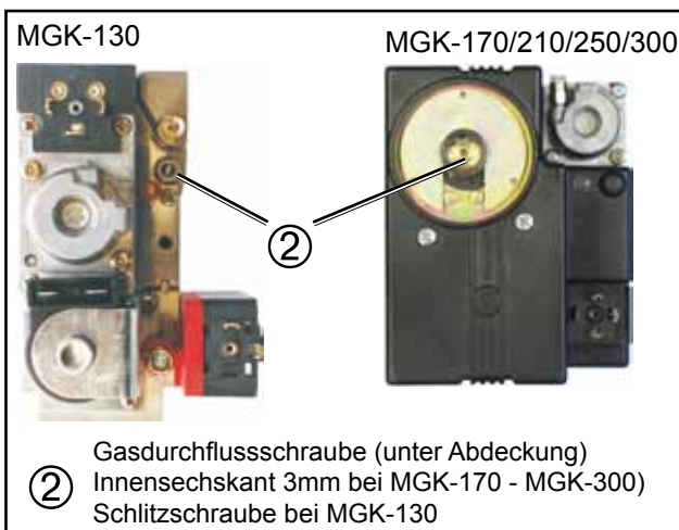
Bild: Gaskombiventil
