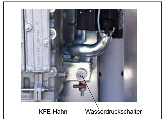
Bild: KFE-Hahn
