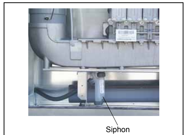
Bild: Siphon
