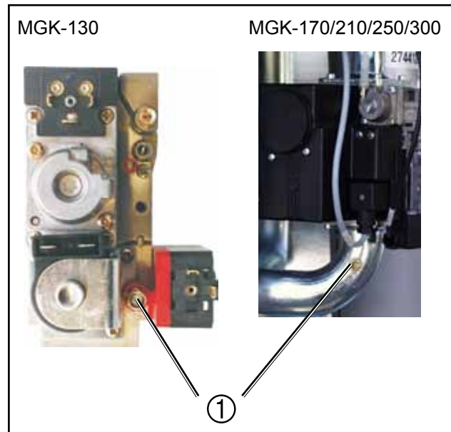
Bild: Messnippel zum Überprüfen des Gasanschlussdrucks
