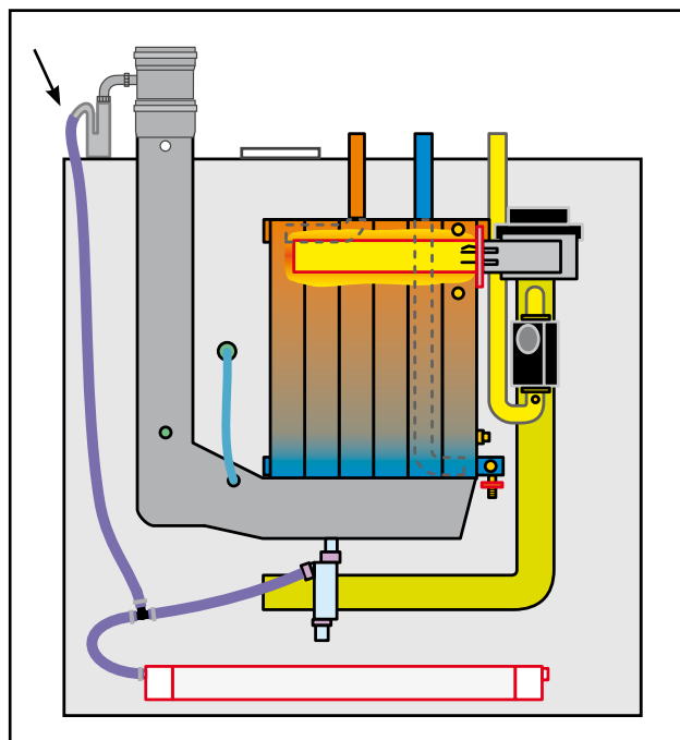
Bild: Kondensatschlauch
