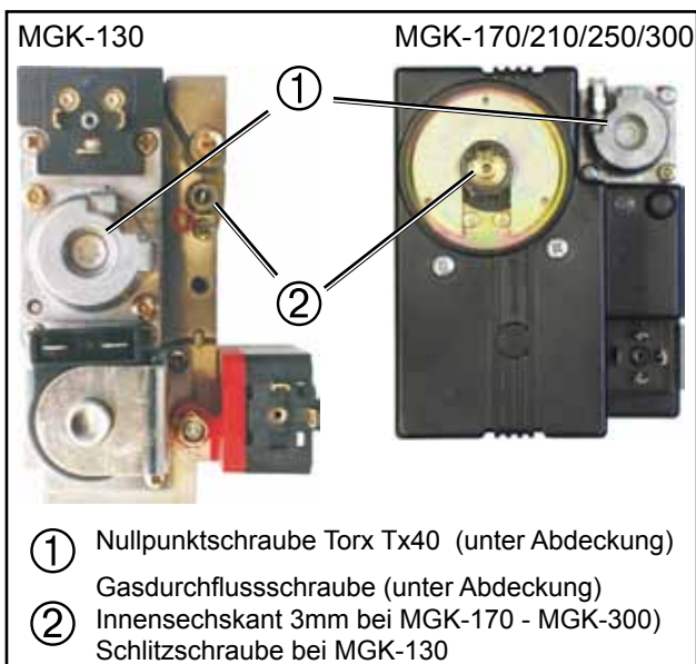
Bild: Gaskombiventil
